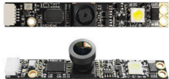
HDF720P-USB2-V1.0(USB) L*W:60*8mm(镜头可选)
